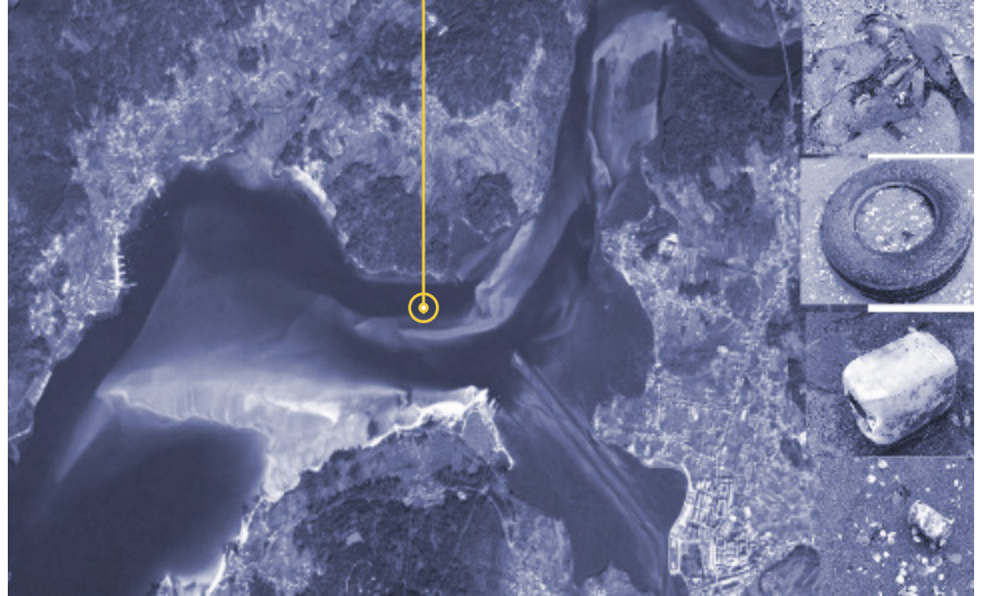
Esteiro do río Tambre e exemplos de lixo mariño atopado.
